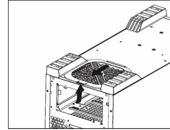
Staubfilter nach hinten rausziehen
