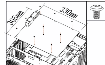
Einbau Mainboard auf dem Träger
