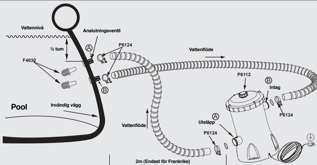
Illustration (inte i skala) av poolen och filterpumpen KOLCHAKA™
